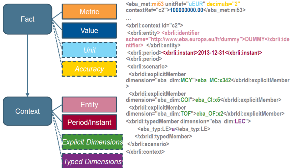
Kuva 3: XBRL-raportin rakenne
